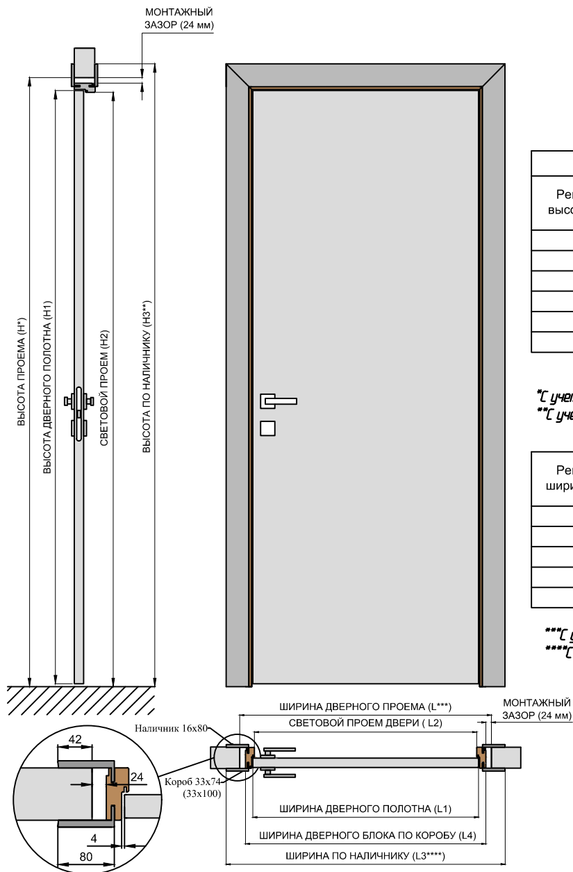
Таблицы соответствия размеров дверных блоков и проемов
